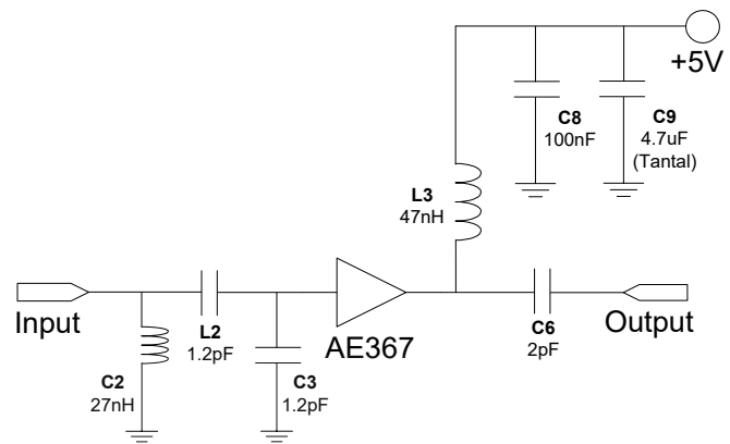
EVB BOM
