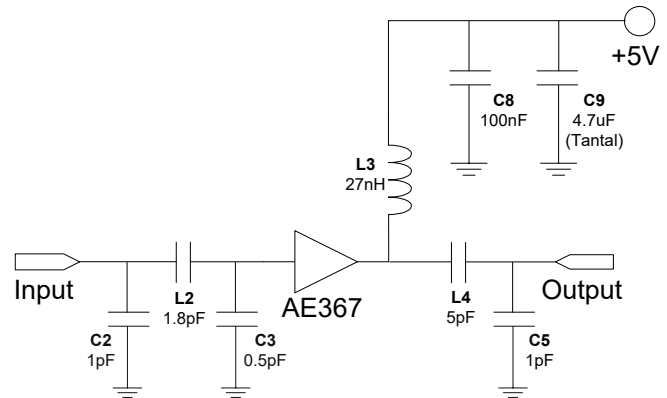
EVB BOM
