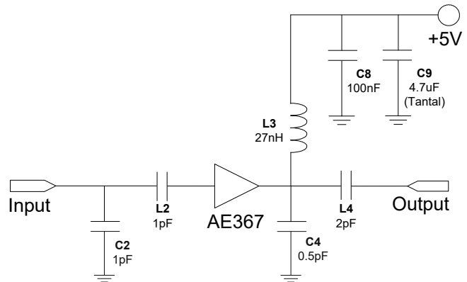
EVB BOM
