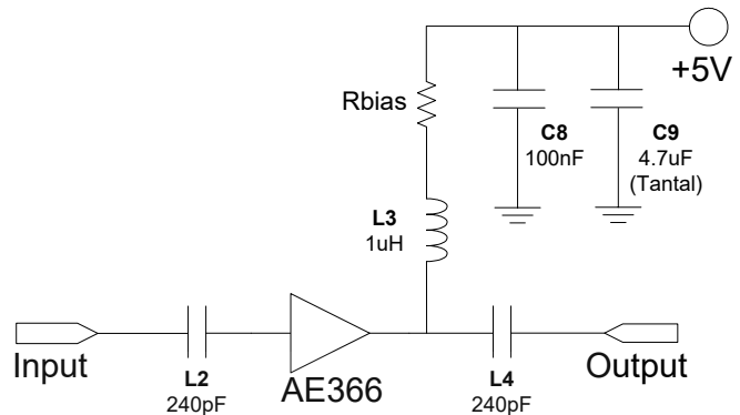
EVB BOM
